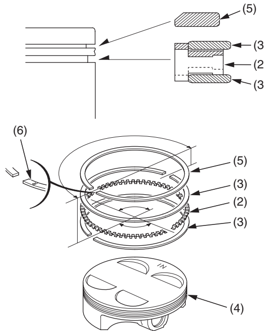
(2) separador (3) rieles laterales (4) pistón
