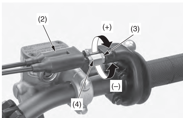
(2) cubierta contra el polvo (3) contratuerca (4) ajustador (+) incrementar (–) reducir
