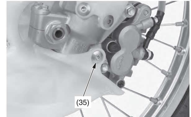
(35) perno de cabeza hueca de la cubierta del disco
