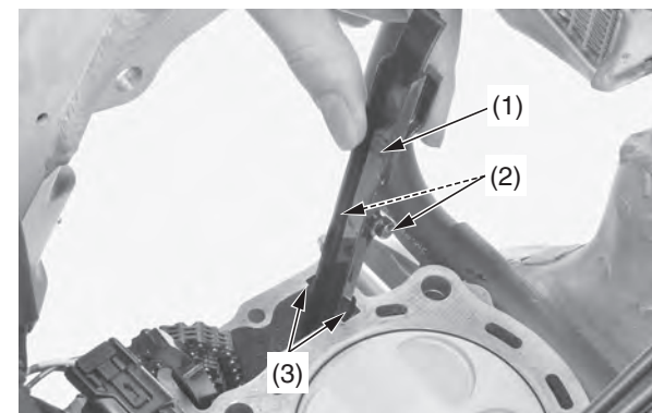
(1) guía de la cadena de levas (2) lengüetas de la guía de la cadena de levas (3) cortes del cilindro
