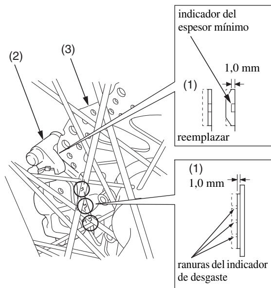
(1) pastillas del freno (2) pinza del freno delantero
