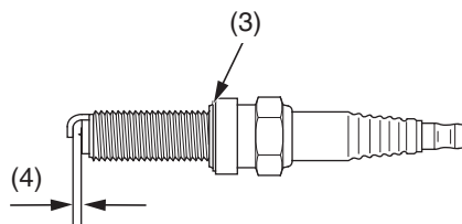
(3) empaquetadura de sellado
