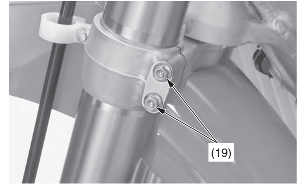
(19) pernos de fijación inferiores del puente de la horquilla
