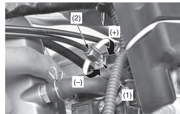
(1) contratuerca (2) ajustador (+) aumentar el juego libre (–) reducir el juego libre
