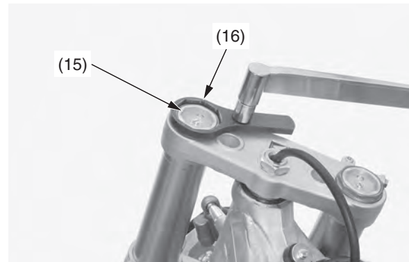
(15) amortiguador de la horquilla (16) llave de contratuerzas
