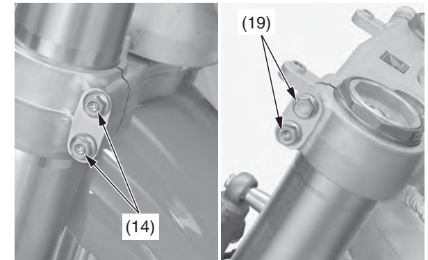
(14) pernos de fijación inferiores del puente de la horquilla (19) pernos de fijación superiores del puente de la horquilla
