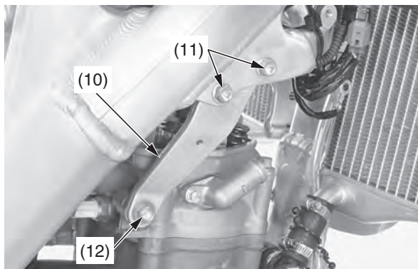
(9) placa izquierda del soporte de la culata (10) placa derecha del soporte de la culata (11) pernos de la placa del soporte de la culata (12) pernos del soporte de la culata
