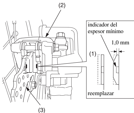
(1) pastillas del freno (2) pinza del freno trasero
