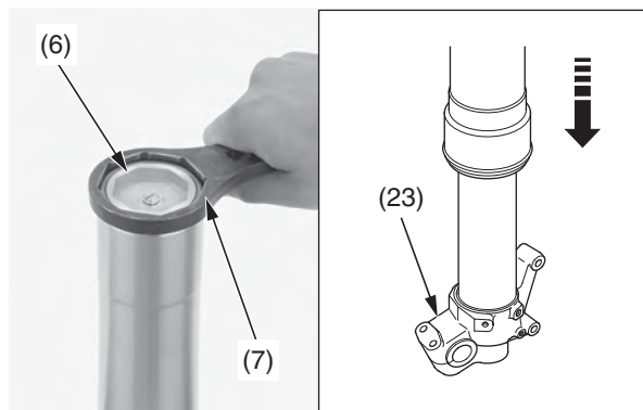
(6) amortiguador de la horquilla (23) soporte del eje (7) llave de contratuerca
