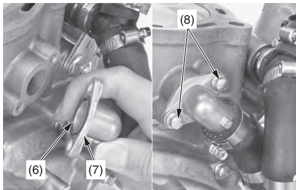
(6) junta tórica (nueva) (7) junta de la manguera de agua (8) pernos
