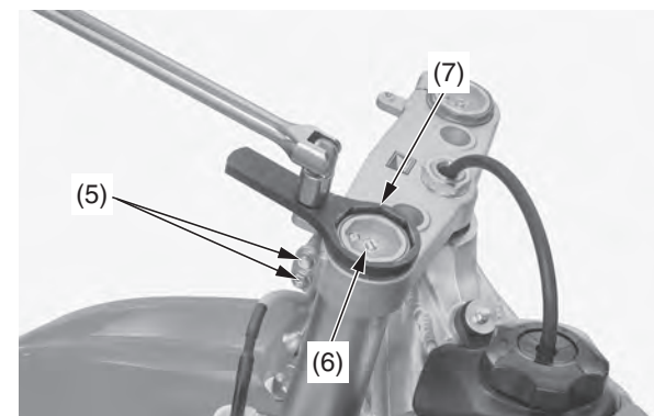
(5) pernos de fijación superiores del puente de la horquilla (6) amortiguador de la horquilla (7) llave de contratuerzas
