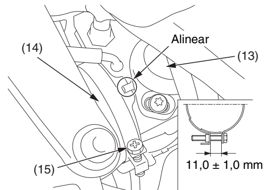
(13) cuerpo del acelerador (14) aislador (15) tornillo de la banda del aislador
