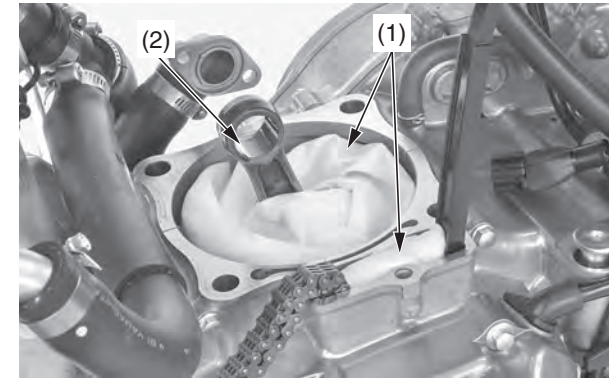
(1) paños de taller (2) pie de la biela
