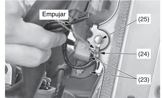
(23) bobina de encendido/soporte (24) cable de toma de tierra (25) perno
