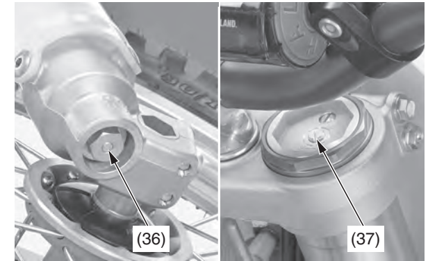
(36) ajustador de la amortiguación de expansión (37) ajustador de la amortiguación de compresión
