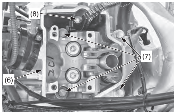
(6) culata (7) arandelas y pernos de la culata (8) perno del cilindro
